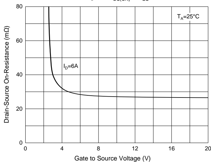
Fig. 4 - R_{DS(ON)} - V_{GS}
